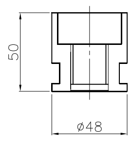
埋設用脚
